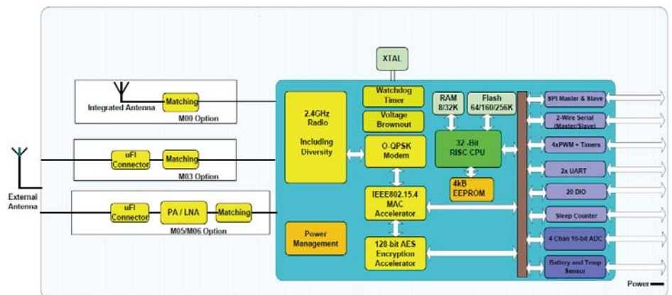
模块结构图
