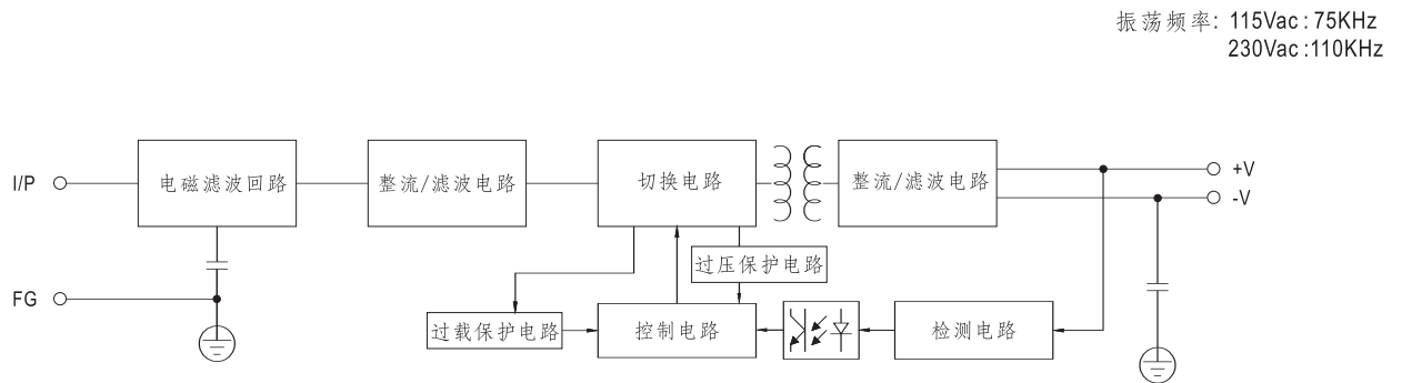
■ 方框图
