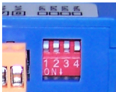
DP4 拨码开关
